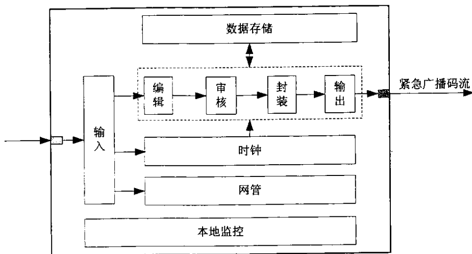
图1 移动多媒体广播紧急广播发生器的功能框图
